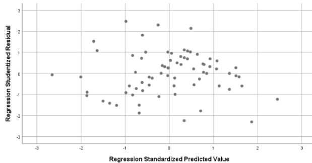
Gambar 1. Grafik Scatterplot
